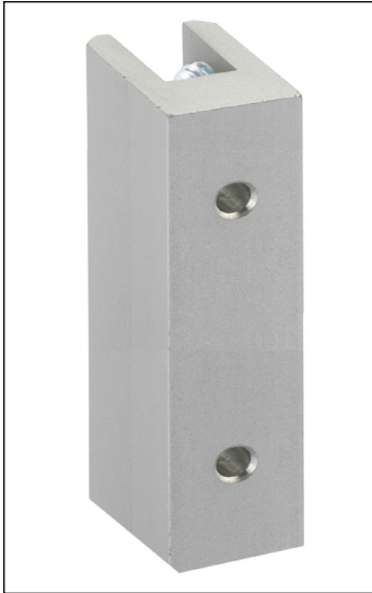
Wandanschluss silber eloxiert mit Stahlklemmschrauben
