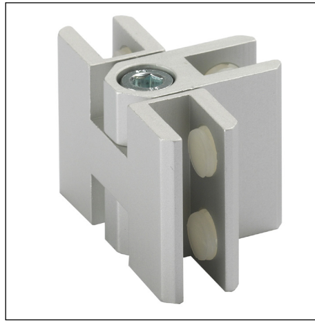
Dreier-Verbinder starr silber eloxiert mit Stahlklemmschrauben
