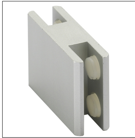
Mittelverbinder silber eloxiert mit Kunststoffklemmschrauben
